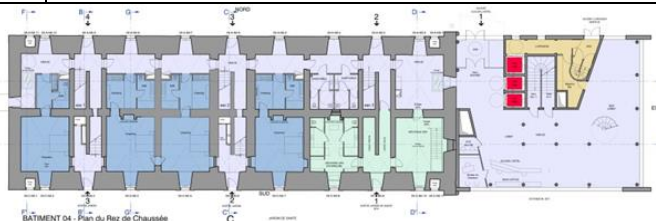
Projet des deux bâtiments des casernes – rez-de-chaussée
