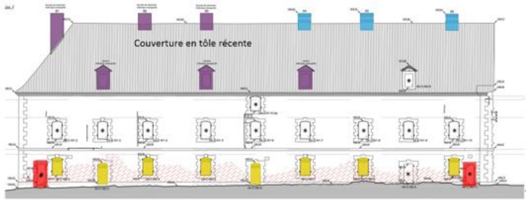
Bâtiment Est des casernes du fort – façade sud
