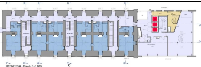
Projet des casernes du fort
