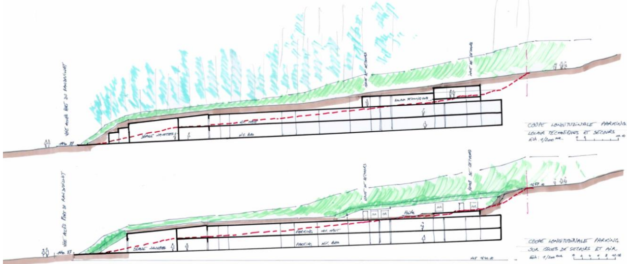
Coupe du projet du parking
