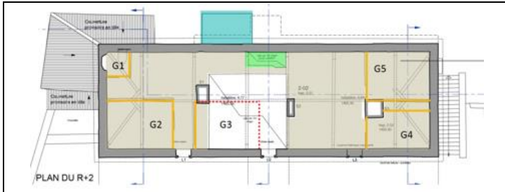
Projet du bâtiment de logis – grenier
