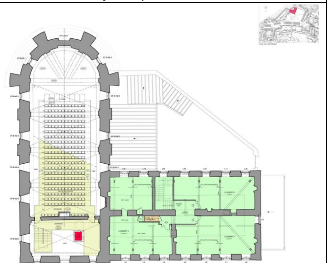
Projet pavillon des officiers – niveau R+2
