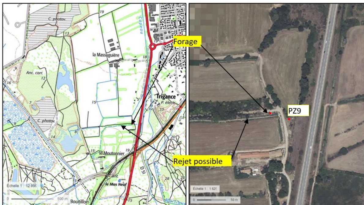
Figure 1 : Plan de localisation, d'accès et d'implantation du chantier
